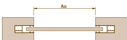
MONTAJE A: GUÍA EMBUTIDA
